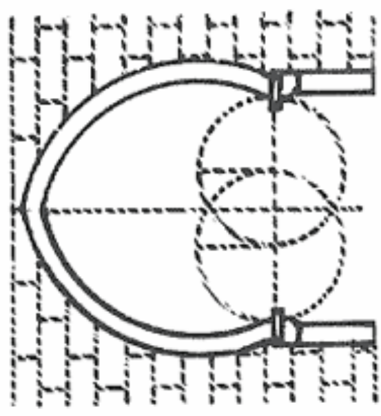
Arco tumbido.
