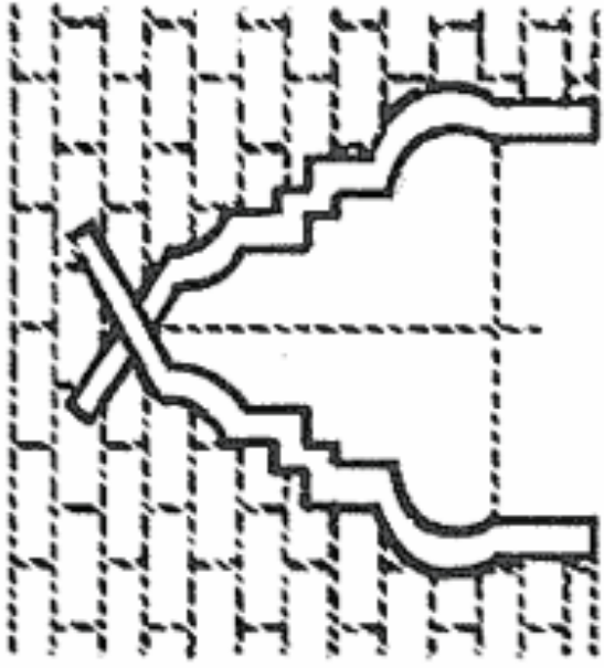
Arco mixtilíneo.
